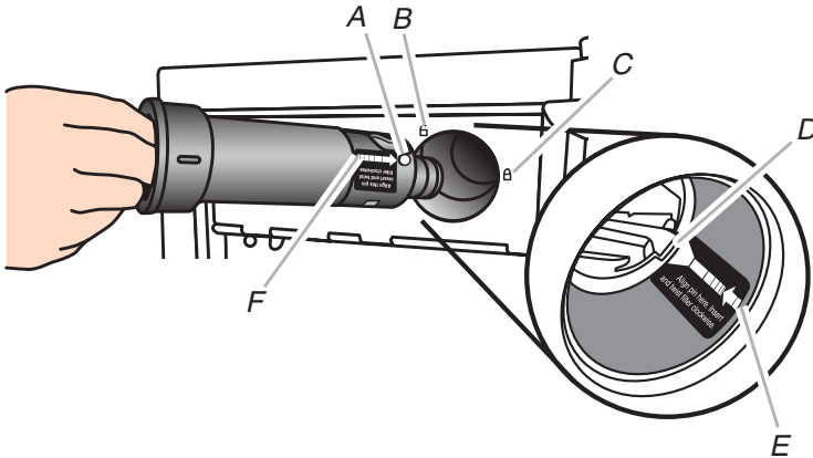
A. Clavija de alineación B. Símbolo de desbloqueado C. Símbolo de bloqueo D. Muesca dentro de alojamiento de control E. Flecha apuntando a muesca F. Flecha apuntando a pasador de alineación
