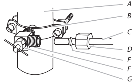
A. Tubería de agua fría B. Abrazadera para tubería C. Tubería de cobre D. Tuerca de compresión E. Manguito de compresión F. Válvula de cierre G. Tuerca de presión
