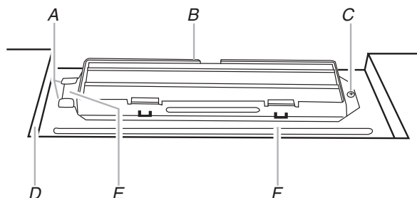
A. Pattes relevées B. Registre C. Vis n° 6 x 3/8 po à tête hexagonale pour tôle D. Ouverture découpée dans l'armoire supérieure E. Patte longue F. Plaque du registre
