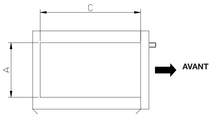
VUE LATÉRALE INTÉRIEURE DE LA CAVITÉ
