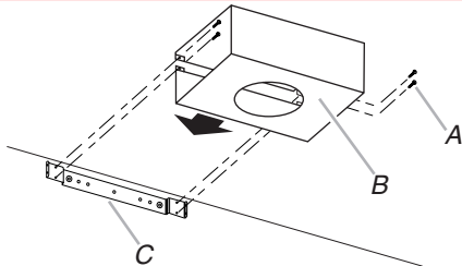
A. Tornillos para el ensamblaje B. Desviador de aire C. Soporte de la cubierta del ducto
