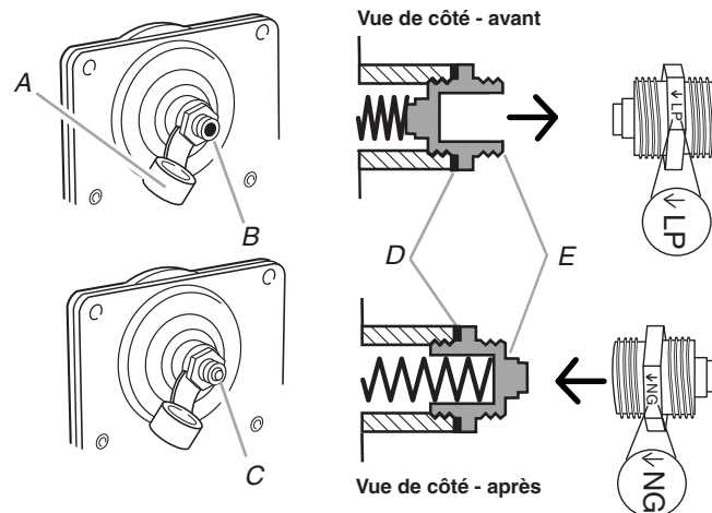
A. Capuchon en plastique B. Capuchon du détendeur; extrémité creuse ouverte vers l'extérieur C. Capuchon du détendeur; extrémité borgne vers l'extérieur D. Rondelle E. Capuchon du détendeur
