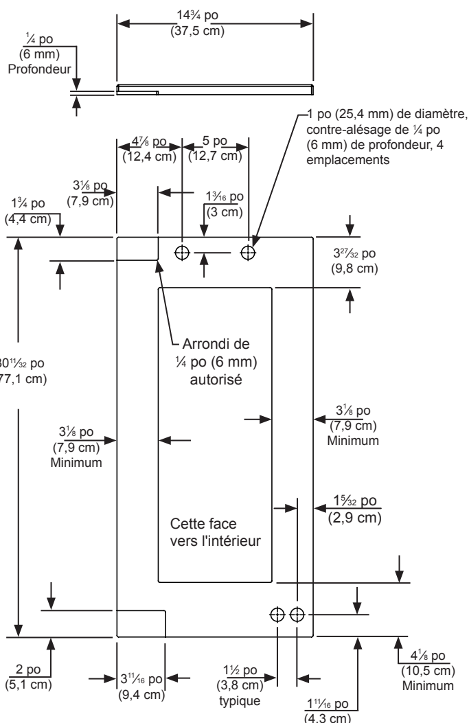
Figure 17 Porte à charnières à droite Appareil de largeur 15 po (38,1 cm)
