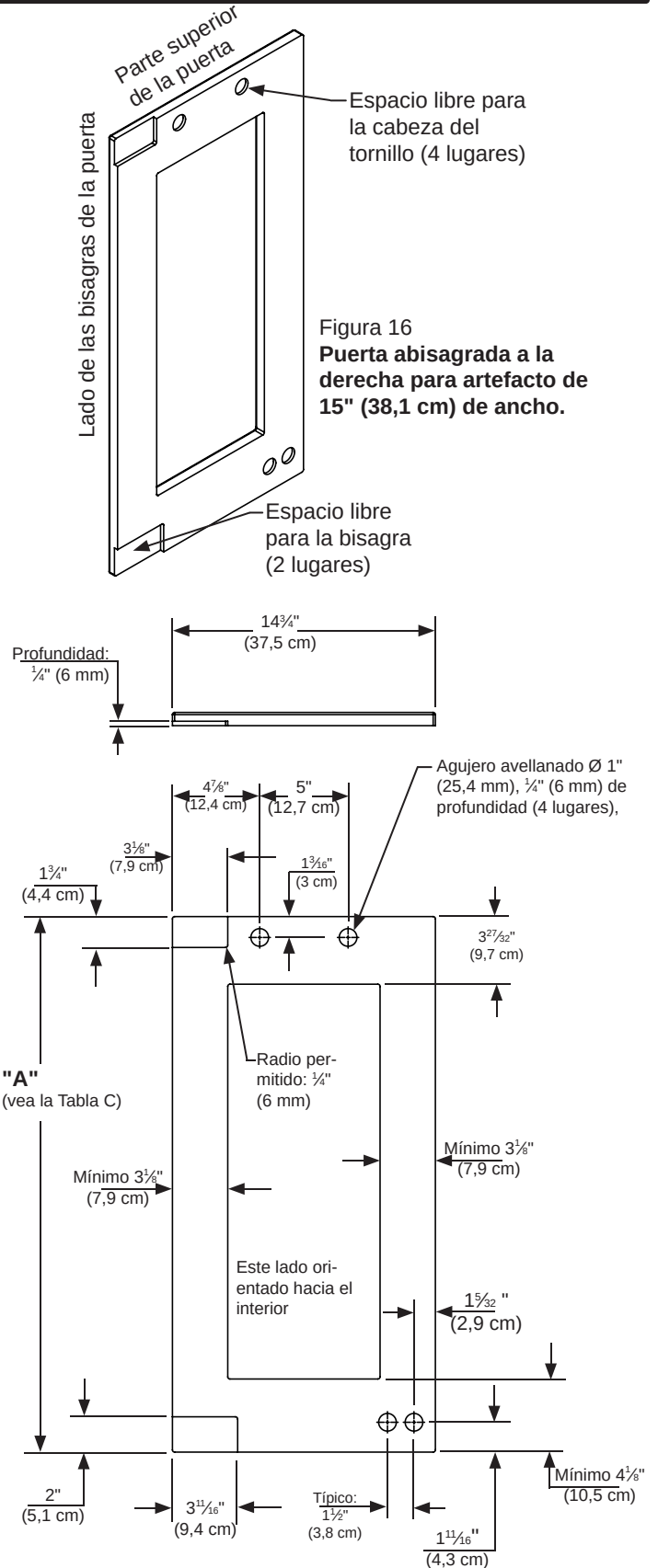
Figura 17 Puerta abisagrada a la derecha para artefacto de 15" (38,1 cm) de ancho.
