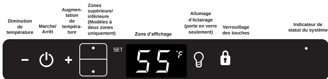
Figure 10 Commandes électroniques
