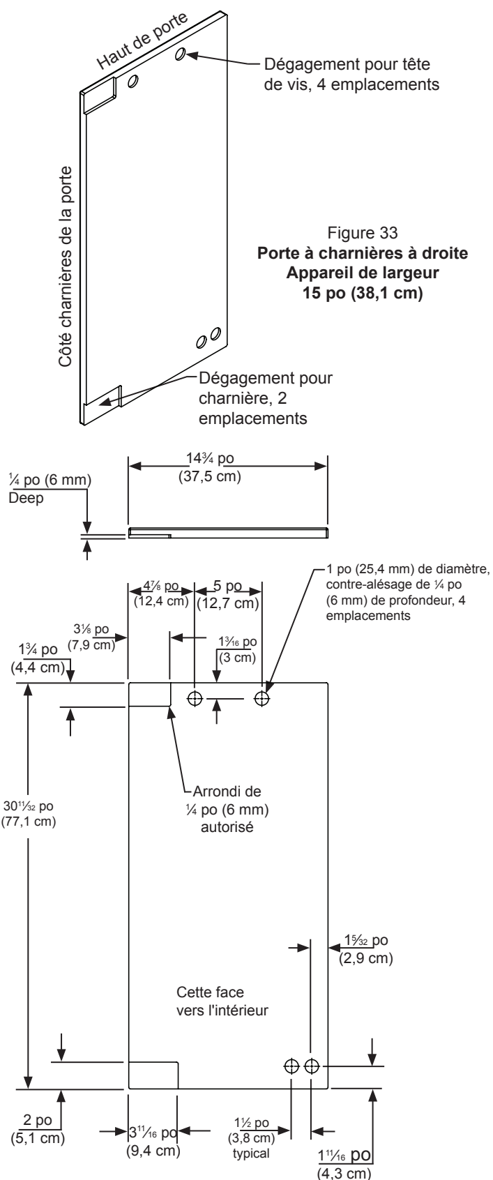
Figure 34 Porte à charnières à droite Appareil de largeur 15 po (38,1 cm)
