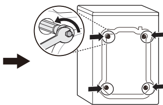
Déballage et retrait des boulons d'expédition
