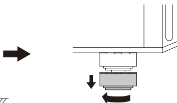
Nivellement de la laveuse
