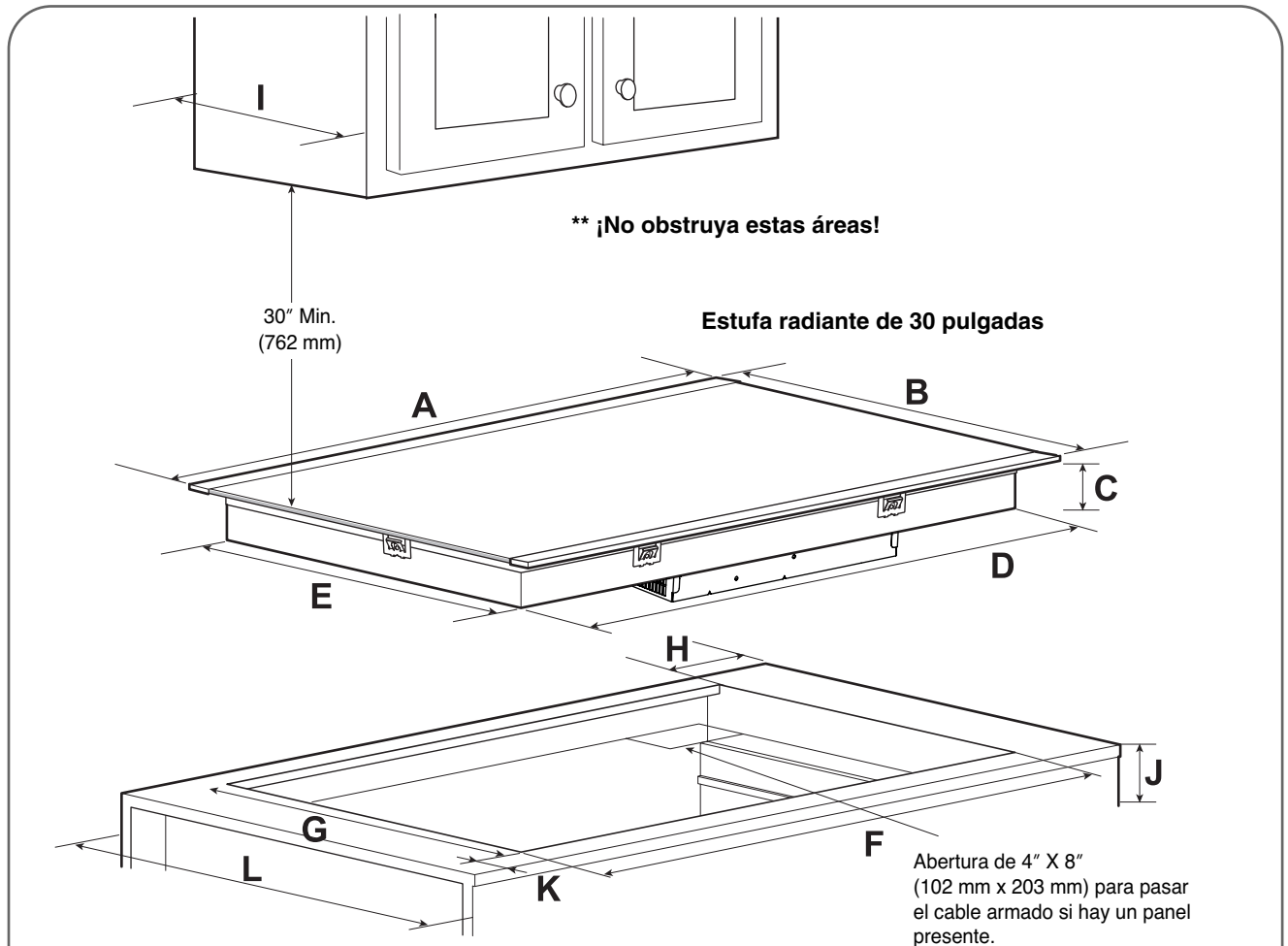
Estufa radiante LSCE305ST
