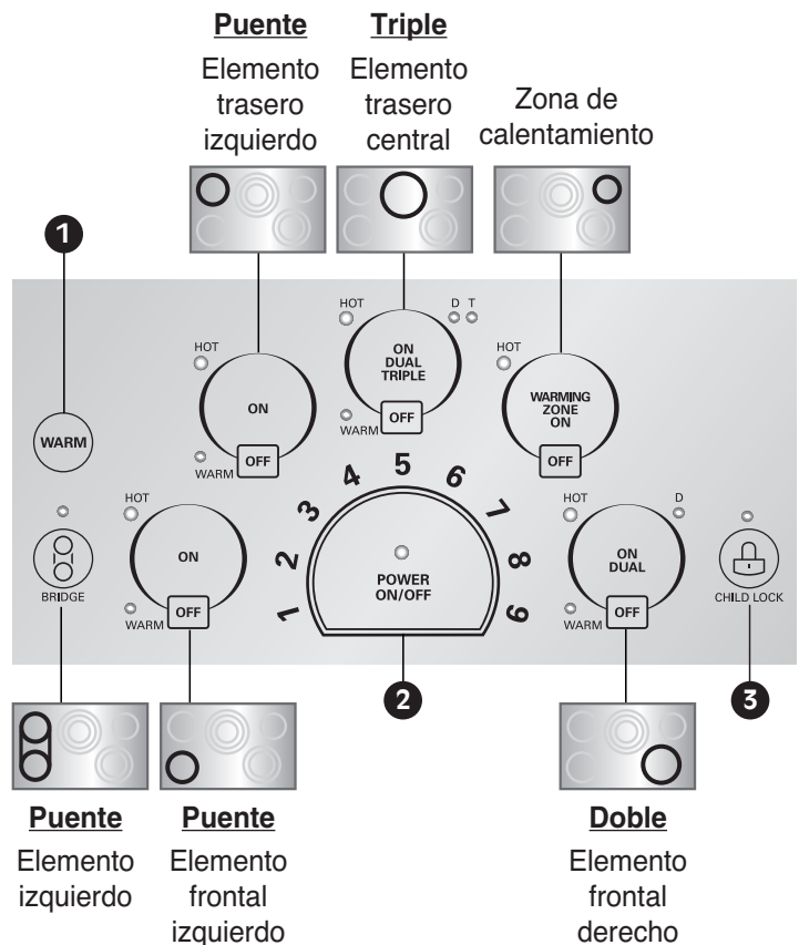
Estufa radiante LSCE365ST
