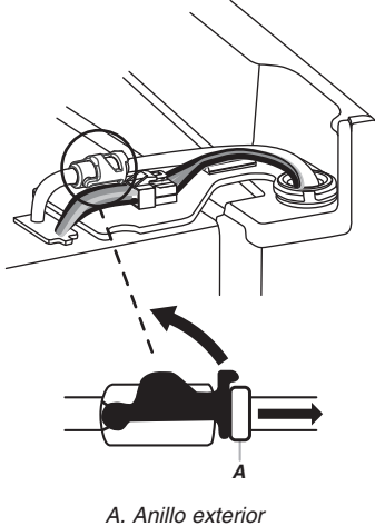
A. Anillo exterior
