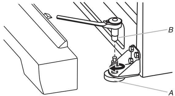
A. Pata con freno B. Llave de hexagonal de 1/4"
