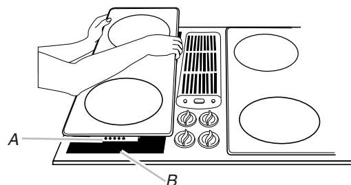
A. Prise mâle du module amovible B. Prise femelle
