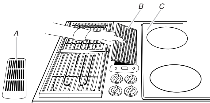
A. Grille de ventilation (précédemment retirée) B. Filtre à graisse amovible C. Module amovible de plaques chauffantes
