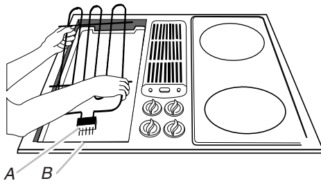
A. Prise mâle de l'élément du grill B. Prise femelle
