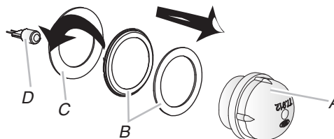
A. Protège-ampoule B. Joints C. Anneau métallique D. Ampoule halogène
