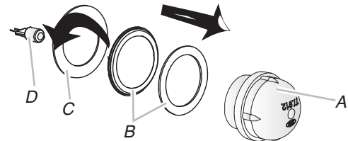
A. Glass cap C. Metal ring B. Seals D. Halogen bulb
