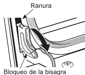
Empuje los bloqueos de la bisagra hacia abajo para desbloquear
