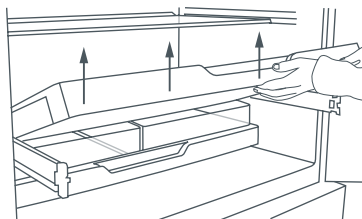
Fig.33 Retrait du plateau
