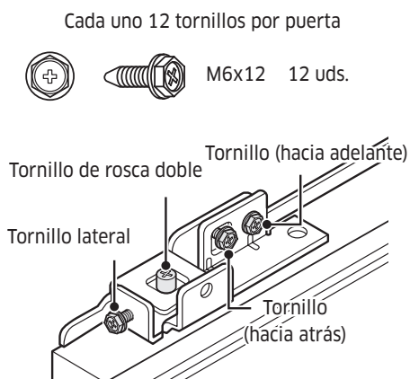
Mecanismo de ajuste de panel
